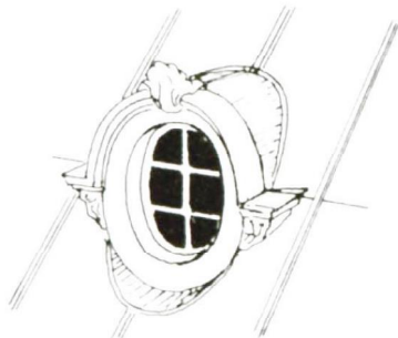
lucarne dite œil-de-boeuf , habillage en zinc façonné
